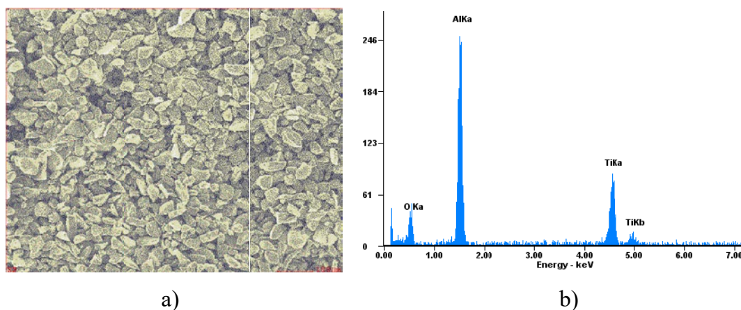
Fig. 2. \text{Al}_2\text{O}_3 - 13 \text{ TiO}_2 powder: a) (SE) image; b) EDS spectrum
