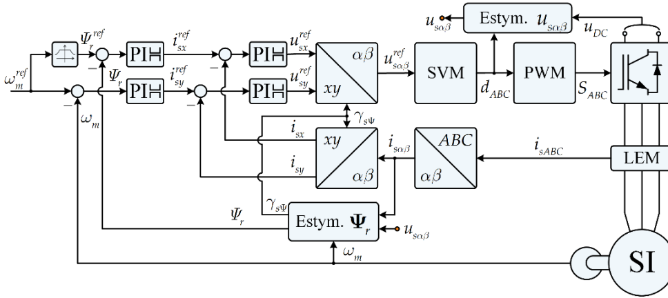
Fig. 4. DFOC scheme.
