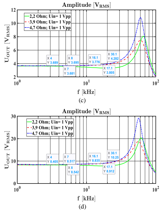
Fig. 6. Amplitude characteristic for (a) TPA 3250 (b) TPA 3251 (c) TPA 3223 (d) TPA 3255
