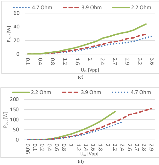
Fig. 5. Output power of the amplifiers (a) TPA 3250 (b) TPA 3251 (c) TPA 3223 (d) TPA 3255
