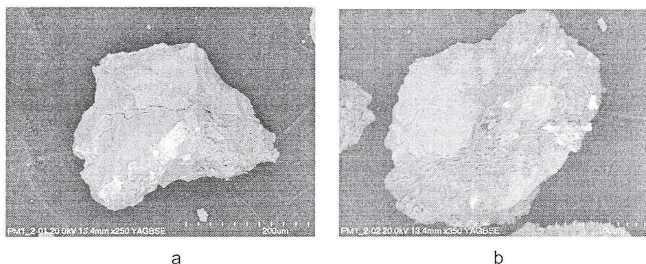
Rys. 4. Frakcja magnetyczna wydzielona z kopaliny ze Sławniowic; a – ziarno kwarcu z wrostkami minerałów żelazistych; b – przerosty ilasto-apatytowe z minerałami REE (jasne fragmenty). SEM
