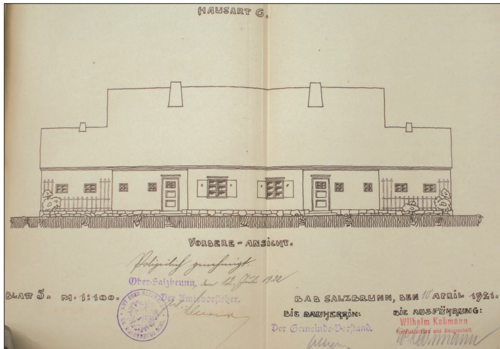
16. Projekt elewacji budynku bliźniaczego na osiedlu na Piaskowej Górze. Opracowany w lokalnym oddziale w Szczawnie w oparciu o budynki typowe „Schlesisches Heim”, projekt. Reprodukacja bez skali. Archiwum m. Szczawna, 65/103, s. 58, Siedlung Gemeinden Ober-Salzbrunn. Hausart 6. , M. 1:100, der Ausführung Wilhelm Kahmann, Bad Salzbrunn 15 April 1921
