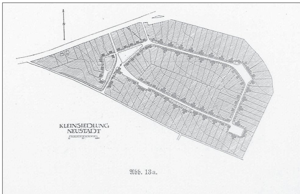
10. Osiedle w Prudniku ( Neustadt ). Projekt. Za: Sonderheft der Schlesischen Landgesellschaft , „Schlesisches Heim”, 1920, b.s.
