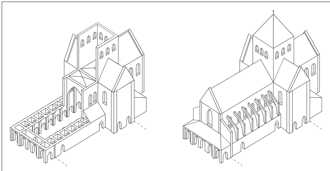
3. T. Węclawowicz: rekonstrukcja faz budowy kościoła w Mogiła w wiekach XIII i XIV (rys. autor) 3. T. Węclawowicz : Reconstruction of the Cistercian church in Mogiła in the thirteenth and fourteenth centuries (drawn by the author)
