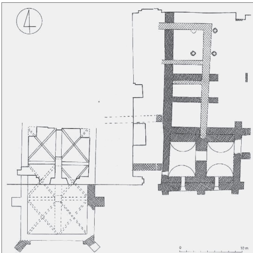
4. B. Kwiatkowska-Kopka: relikty fundamentów klasztoru w Jędrzejowie. Po prawej skrzydło wschodnie, u dołu po lewej refektarz (rys. autorka)
