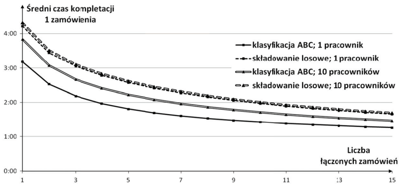
Rysunek 13. Średni czas kompletacji zamówień dla różnej liczby łączonych zamówień i magazynu z 10 alejkami oraz heurystyki return
