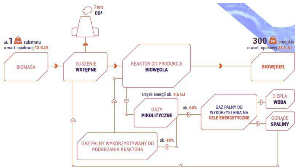
Rys. 3. Przykładowy bilans energetyczny instalacji uwęglania biomasy dla 1 tony substratu o wartości opałowej 13 GJ/Mg (Timex 2018)
