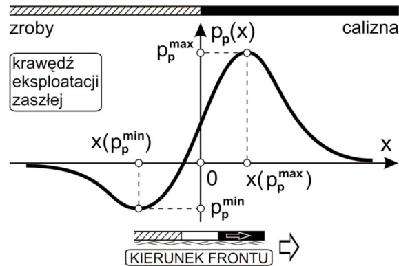
Rys. 3. Schemat naprężeń dodatkowych dla krawędzi (model A)
