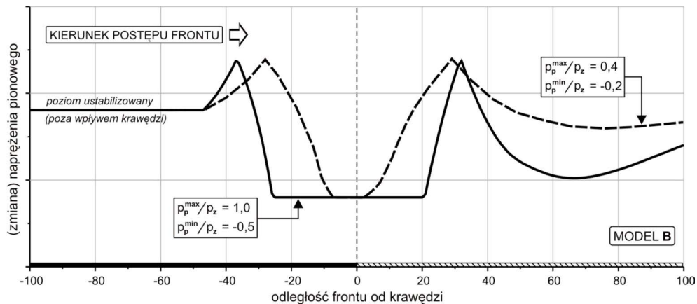
Rys. 8. Rozkład naprężeń na froncie w funkcji dociążenia (model B)
