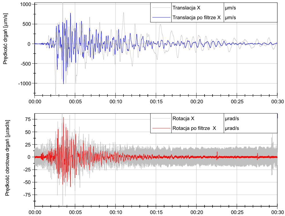
Rys. 5. Sygnał sejsmiczny wstrząsu o energii 1,2 \times 10^7 J przed (zielony) i po filtrowaniu (niebieski)
