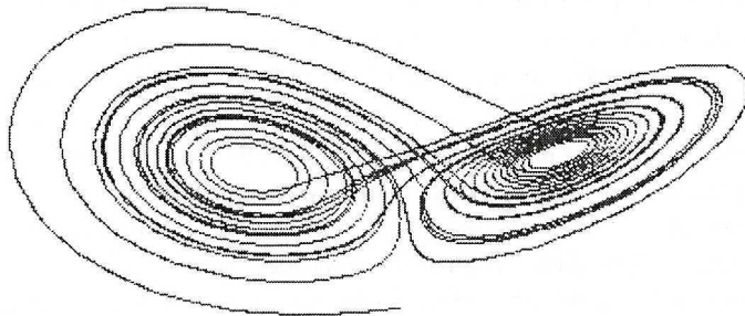
Ryc. 1. Atraktor Lorenza
