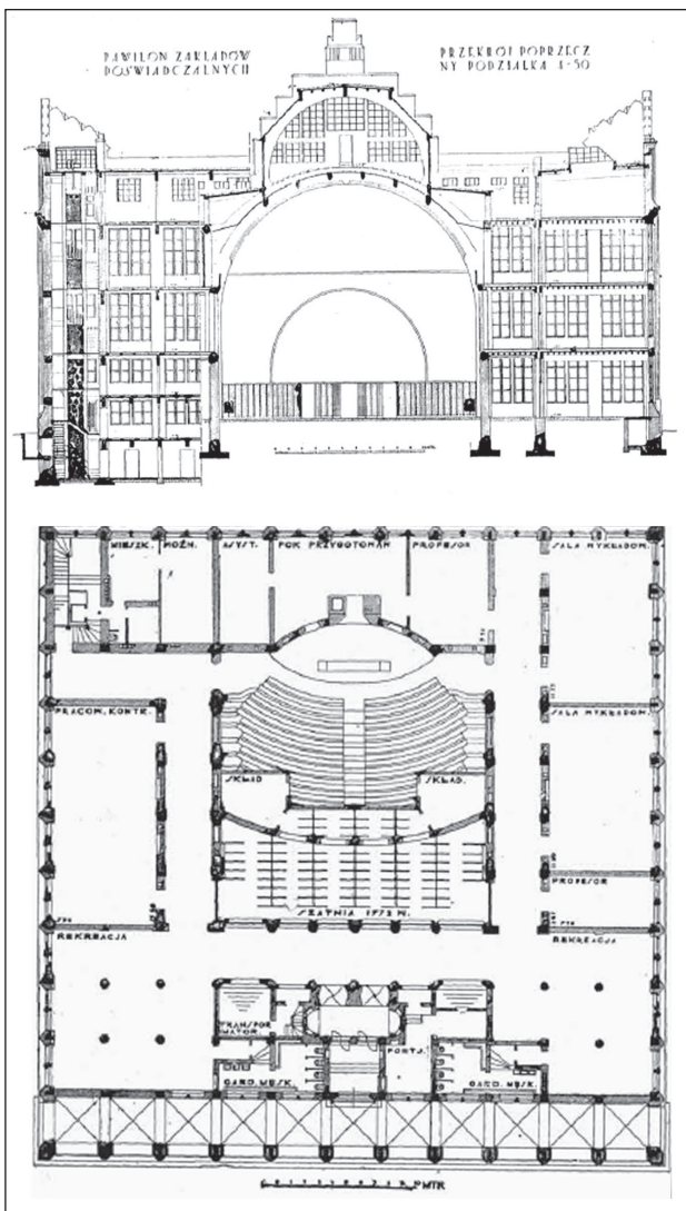
26. Pawilon Doświadczalny Wyższej Szkoły Handlowej, przekrój i rzut parteru, arch. J. Koszczyc-Witkiewicz, 1927. Wg „A i B”, 1927 nr 5, s. 134-135
