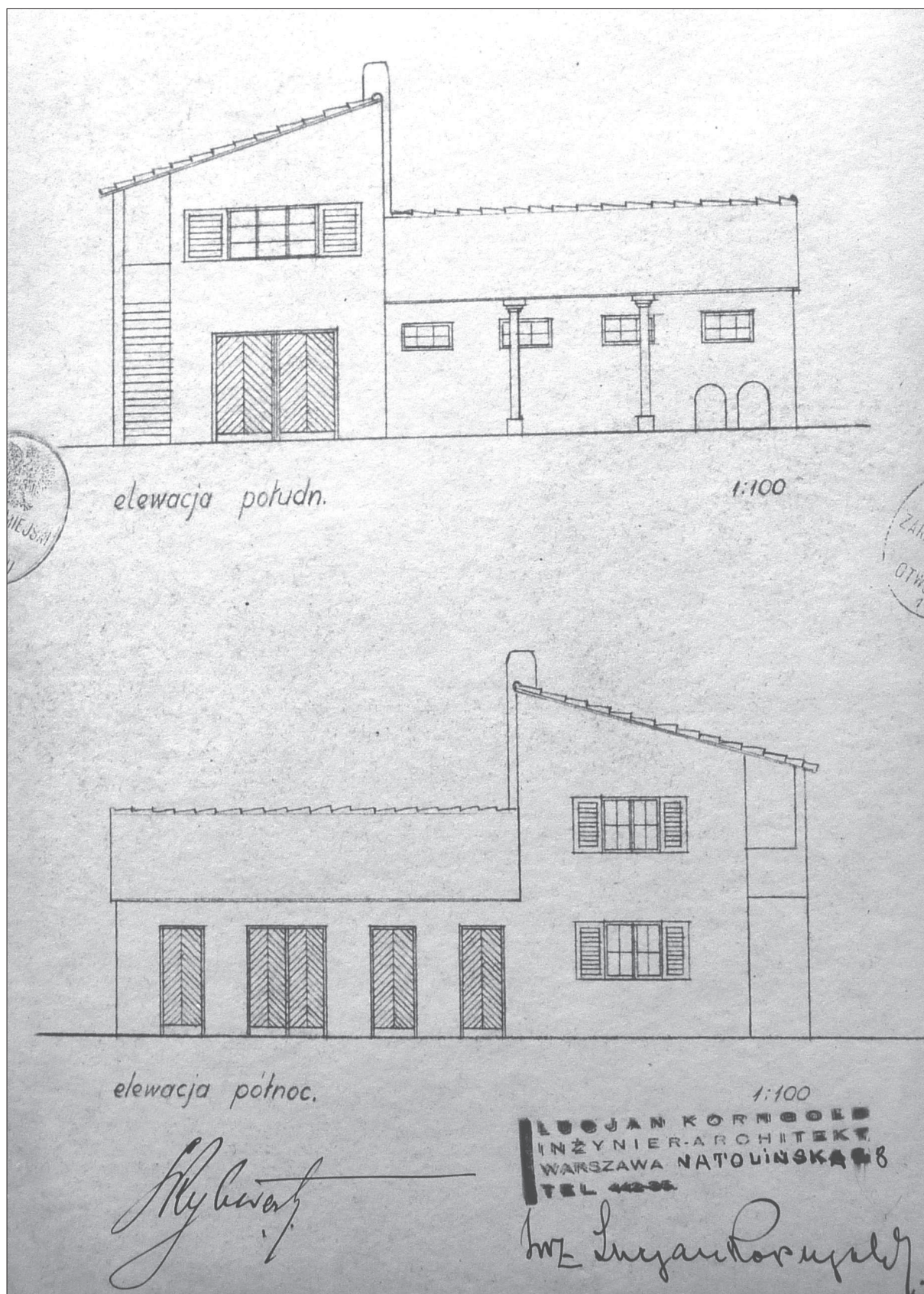
16. L. Korngold, Projekt domu mieszkalnego w Soplicowie k. Otwocka na działkach 97-105, własność S. Rykwert , 8.10.1935 (ul. Myśliwska 2) – elewacja północna i południowa budynku gospodarczego, zrealizowanego ostatecznie wg projektu zamiennego z 1936 r., APW Oddział w Otwocku, AmO, sygn. 4093, k.13
