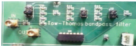
Fig. 10. The actual Tow-Thomas filter.
