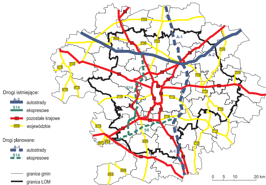
Rys. 1. Sieć głównych dróg kołowych regionu miejskiego Łodzi – stan na 2012 r.
